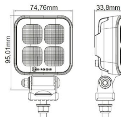
FARETTO DA LAVORO APEX SERIES Compatto — Cavo da 4 metri
