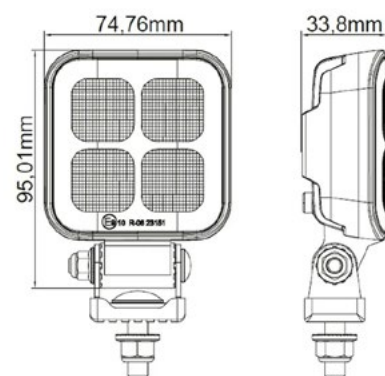
FARETTO DA LAVORO APEX SERIES Compatto — Cavo da 50 cm
