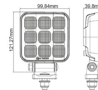
FARETTO DA LAVORO — Apex Series Classico — Cavo da 4 metri
