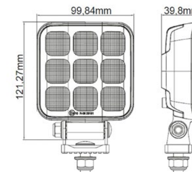
FARETTO DA LAVORO — Apex Series Classico — Cavo da 50 cm
